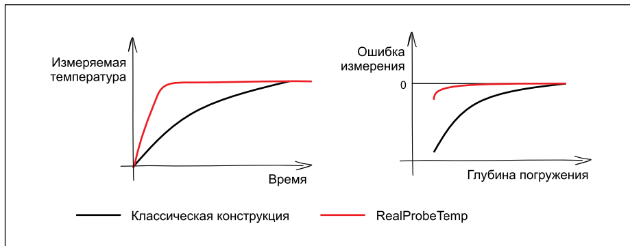
Рис. 12. Сравнение классического исполнения датчика и RealProbeTemp
