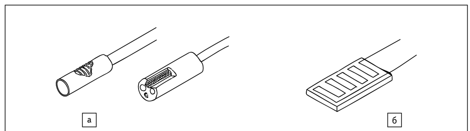
Рис. 5. Конструкции термосопротивлений: а) намоточные; б) тонкопленочные
