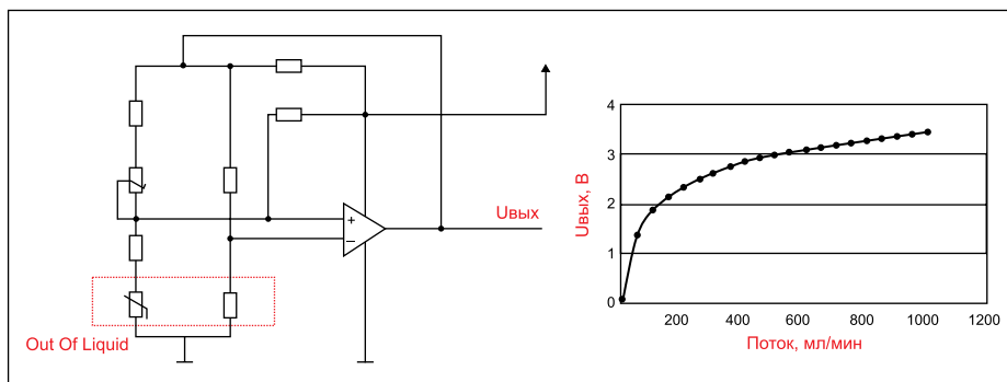
Рис. 15. Пример схемы включения датчика Out Of Liquid и пример выходной характеристики
