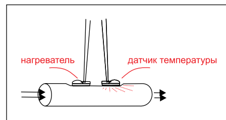
Рис. 14. Конструкция датчика Out Of Liquid
